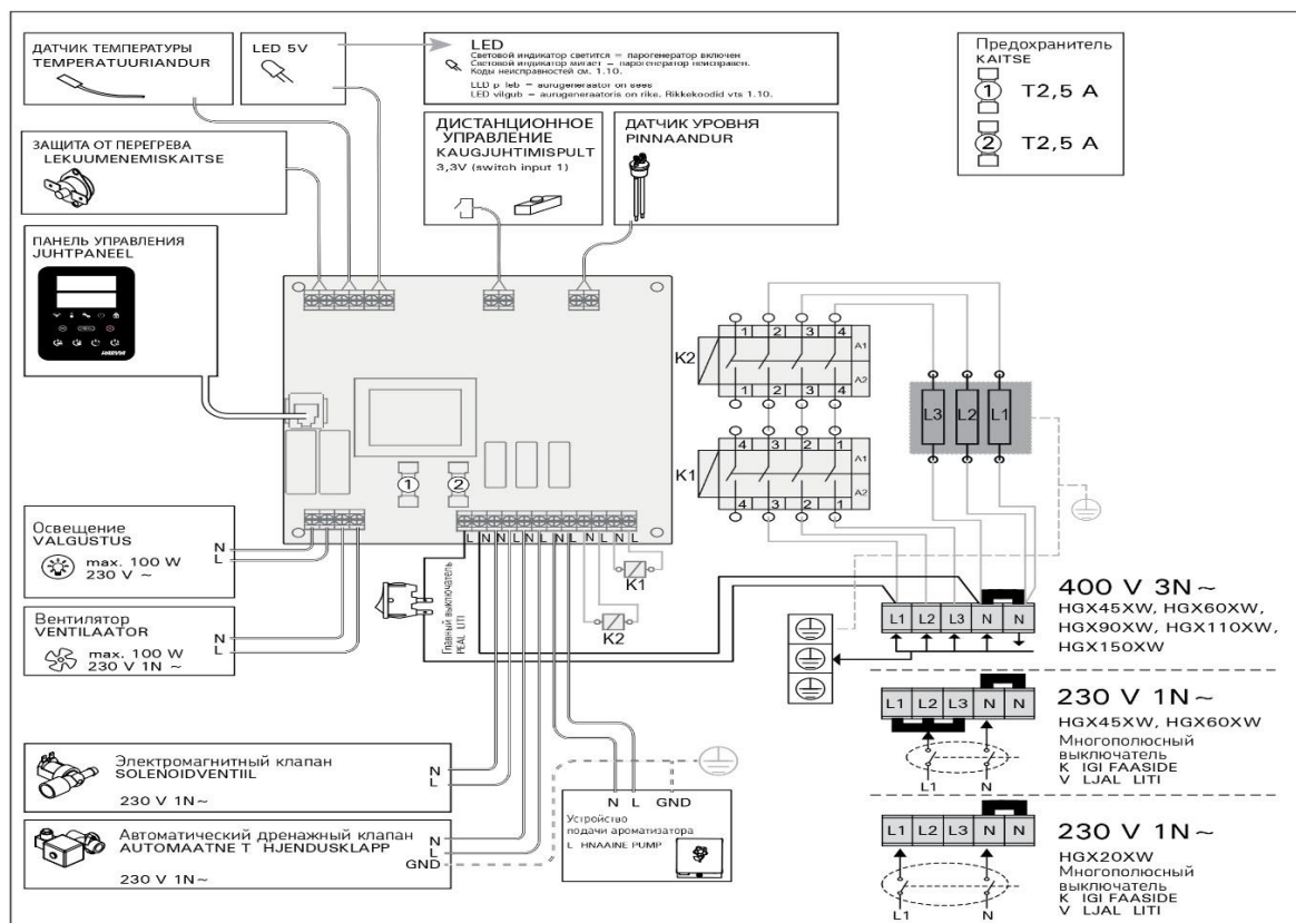
Схема подключения к плате парогенератора.
