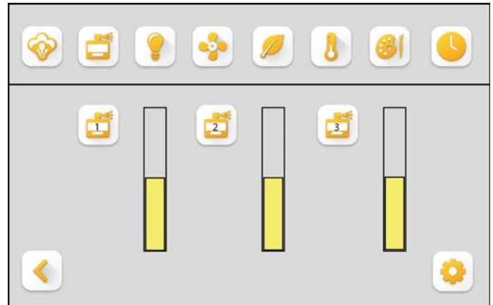
окно при подключении к парогенератору серии HeaterSlim — для главного окна доступно на выбор 3 ароматизатора.
